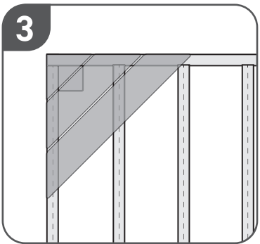
SUBESTRUCTURA DE INSTALACIÓN DIAGONAL 12" en las viguetas máximas del centro. Los ángulos más difíciles pueden requerir un menor espacio entre las vigas.
