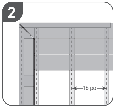
INSTALLATION DE L'INFRASTRUCTURE D'ENCADREMENT Solives de 16 po maximum, centre à centre, auquel s'ajoute un support pour la structure d'encadrement (12 po centre à centre pour les applications commerciales)
