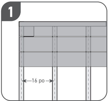
INSTALLATION DE L'INFRASTRUCTURE DE BASE 16 po Solives de 16 po maximum, centre à centre (12 po au centre pour les applications commerciales)
